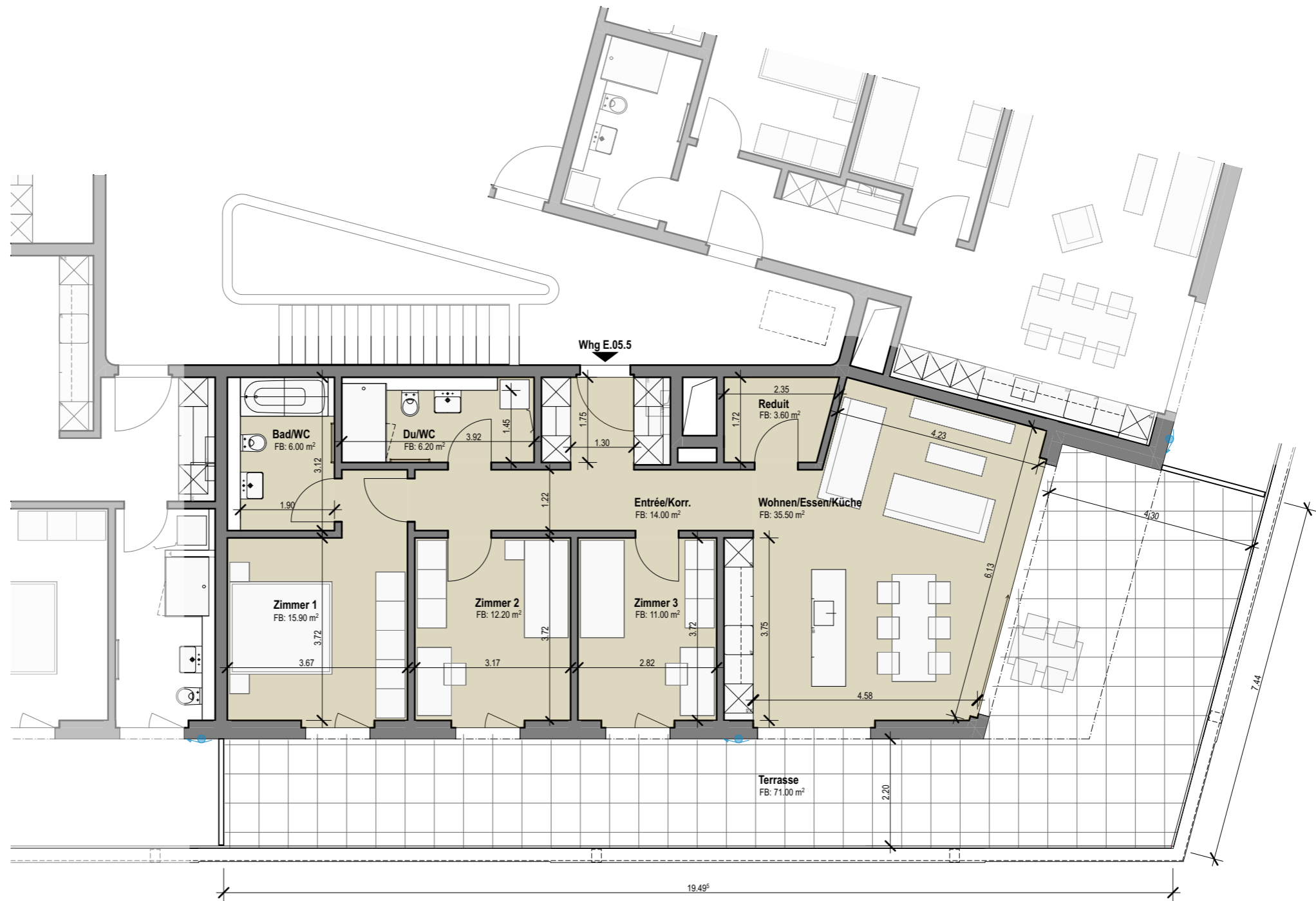
Grundriss Att., Mst. 1:100
