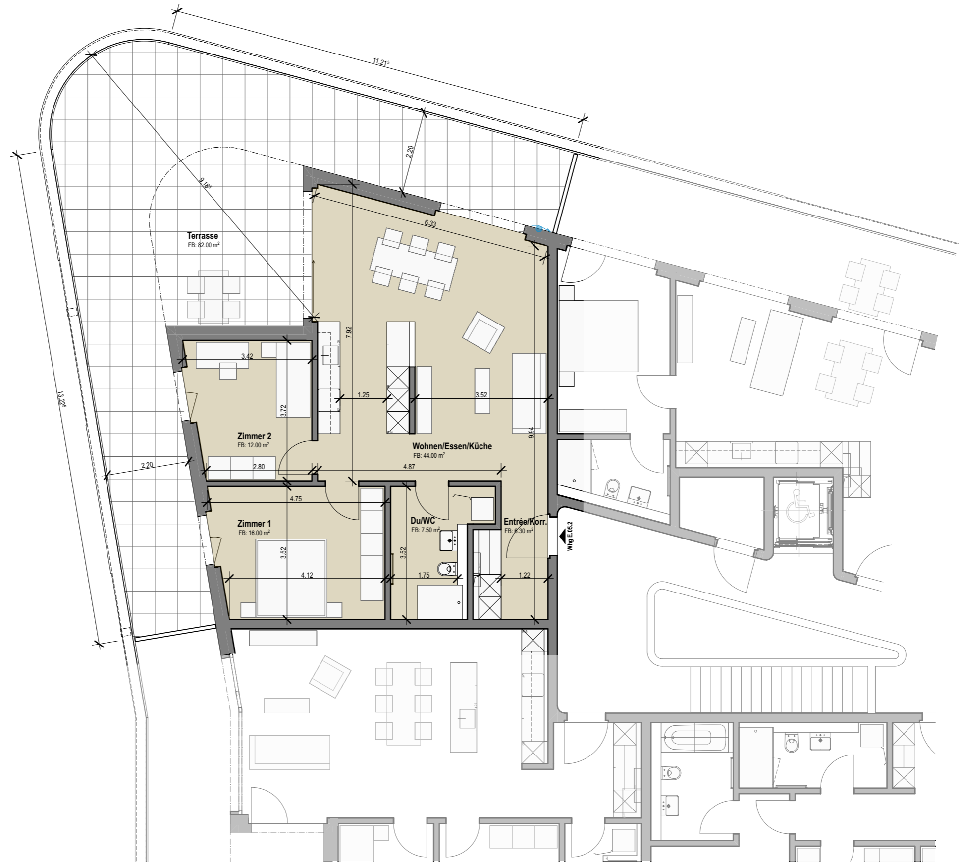
Grundriss Att., Mst. 1:100
