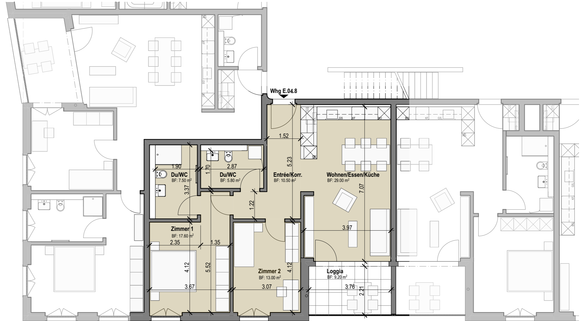
Grundriss 4.OG, Mst. 1:100
