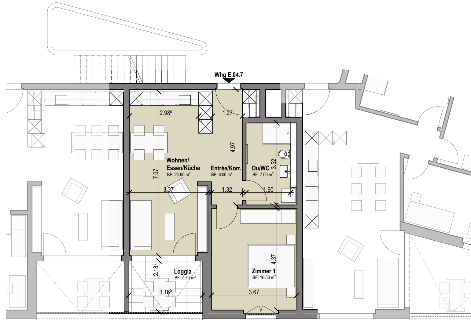
Grundriss 4.OG, Mst. 1:100
