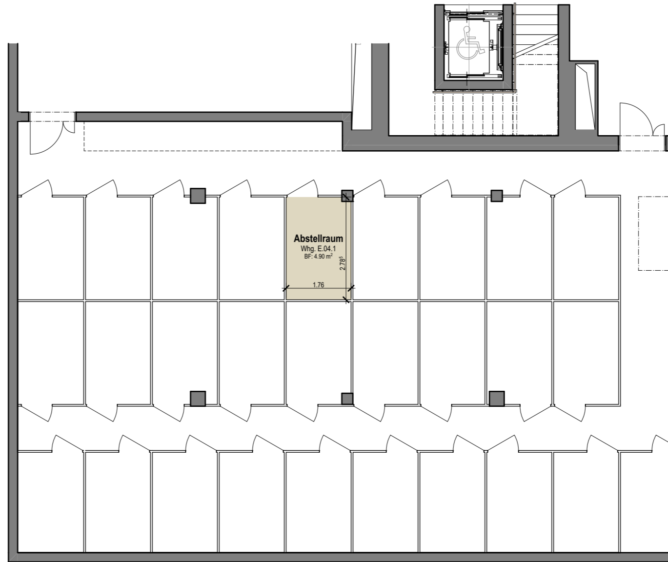
Grundriss -2.UG, Mst. 1:100
