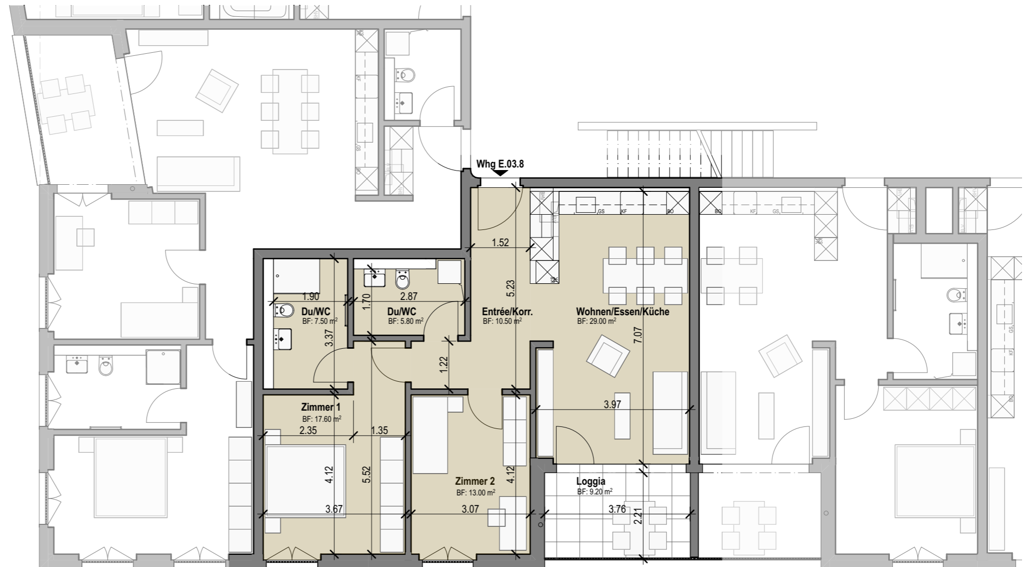
Grundriss 3.OG, Mst. 1:100
