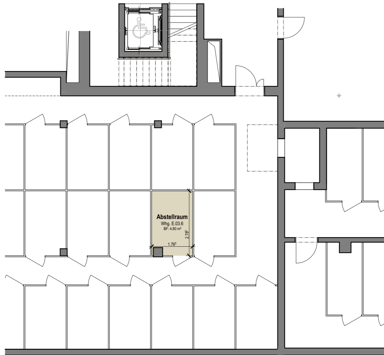
Grundriss -2.UG, Mst. 1:100
