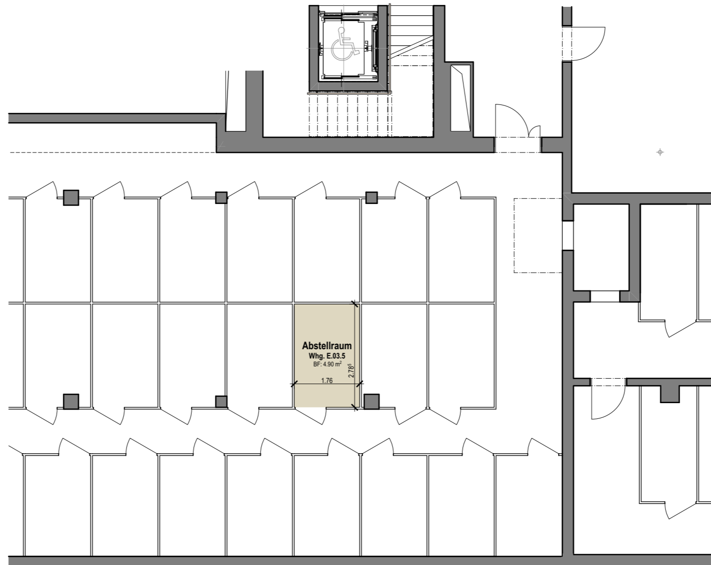
Grundriss -2.UG, Mst. 1:100
