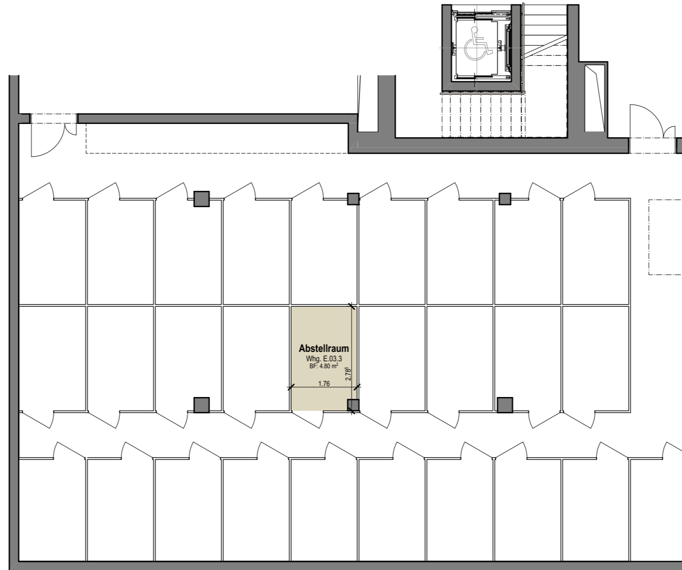
Grundriss -2.UG, Mst. 1:100
