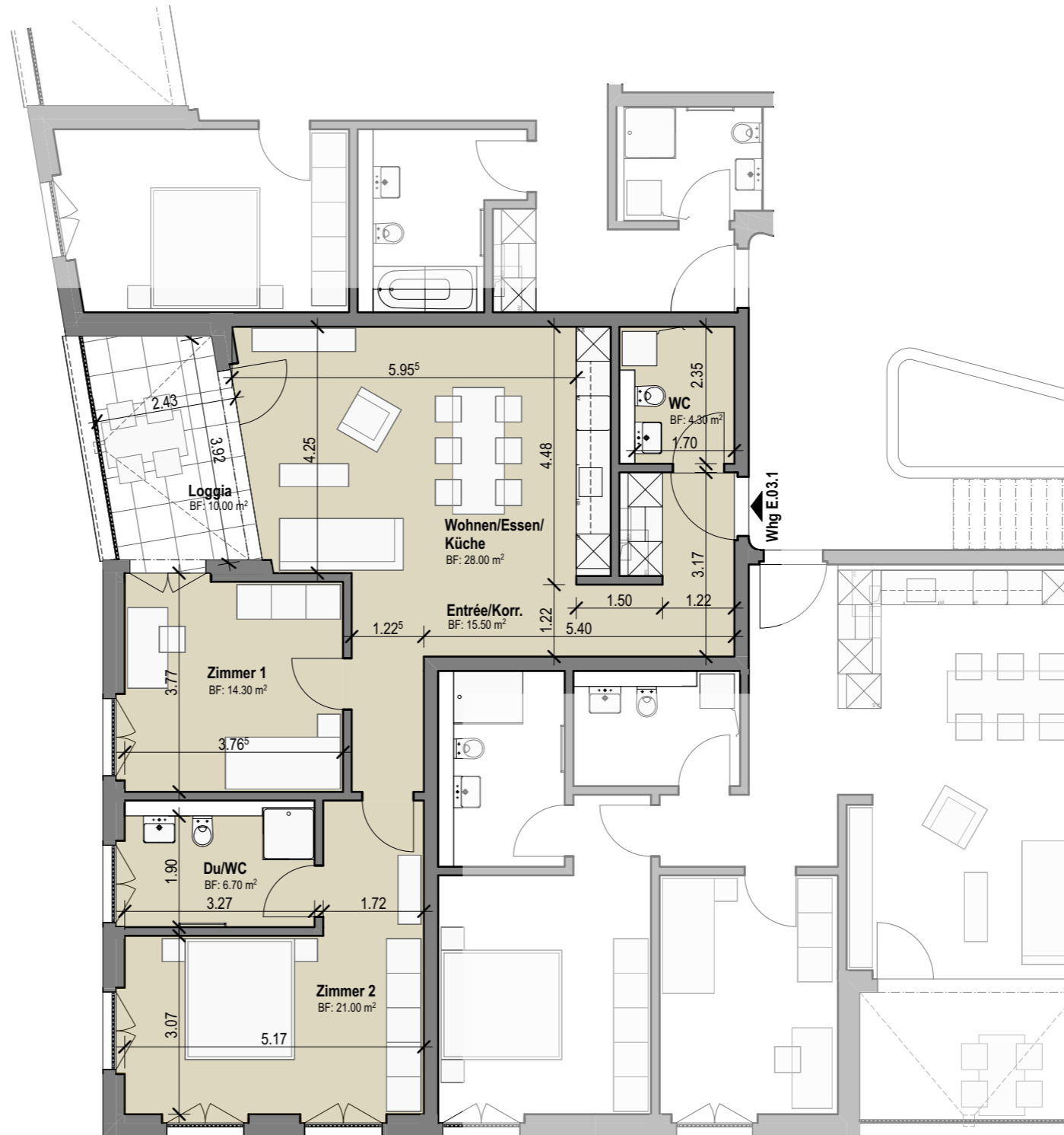
Grundriss 3.OG, Mst. 1:100
