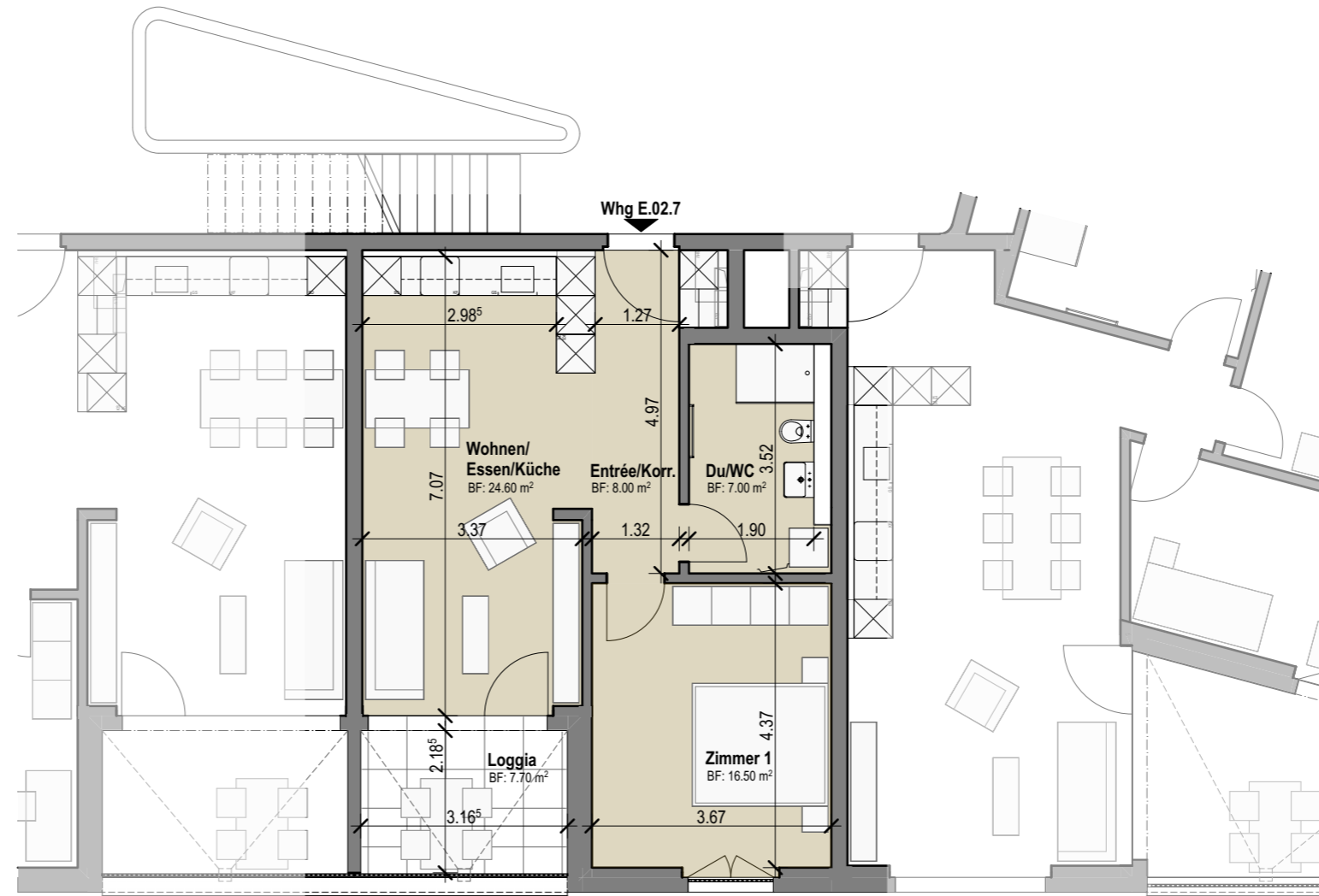
Grundriss 2.OG, Mst. 1:100
