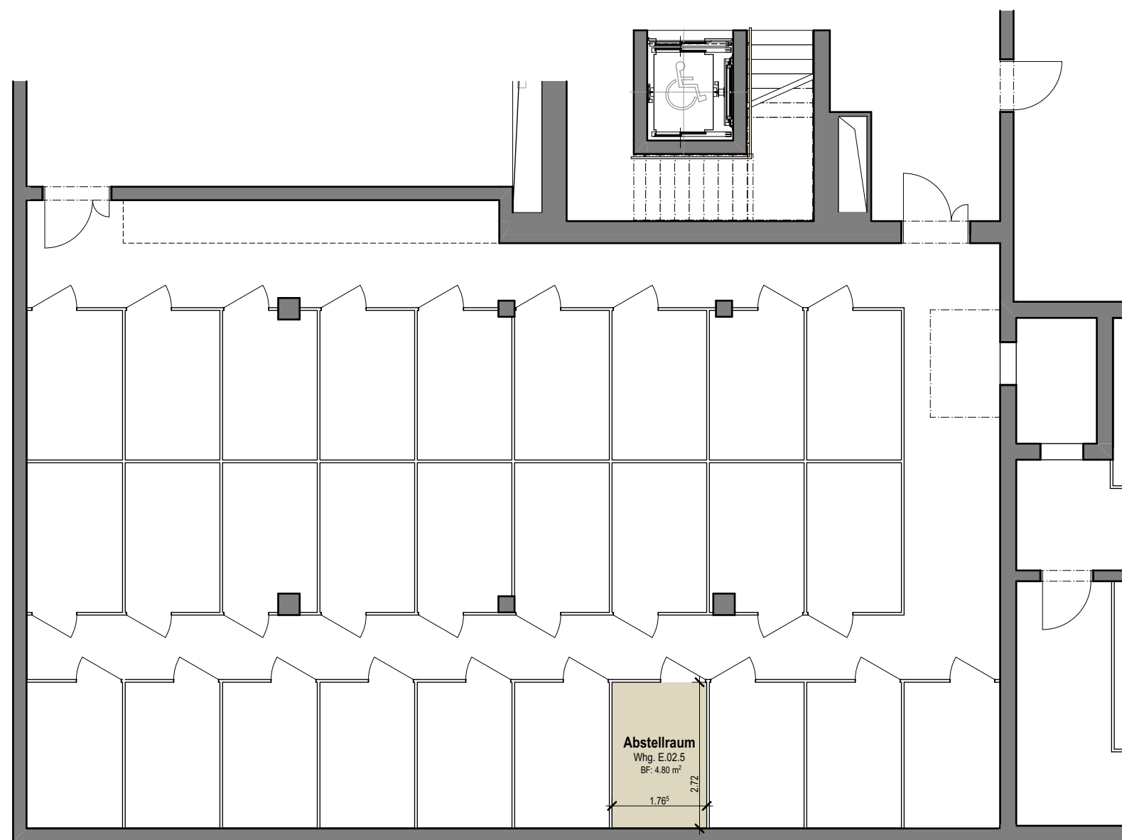
Grundriss -2.UG, Mst. 1:100
