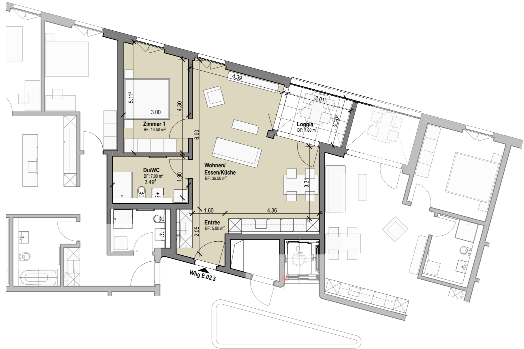
Grundriss 2.OG, Mst. 1:100
