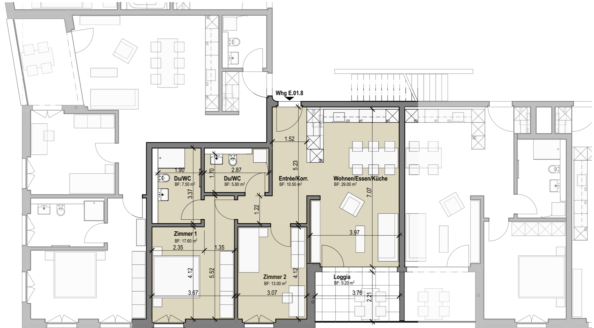
Grundriss 1.OG, Mst. 1:100
