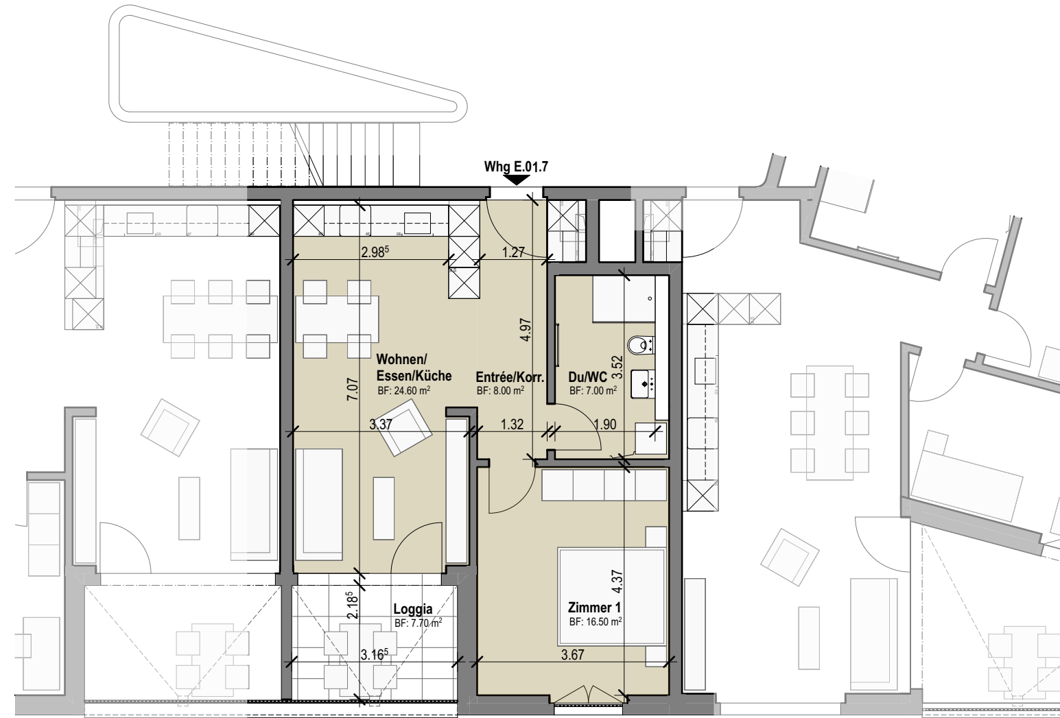
Grundriss 1.OG, Mst. 1:100
